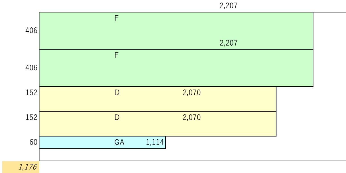
合板3 19mm厚
